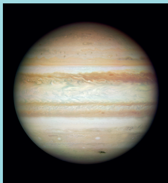
Юпитер
