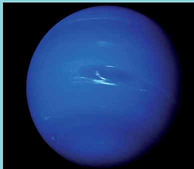
Нептун
