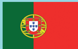
Португалие
