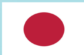
Японие
