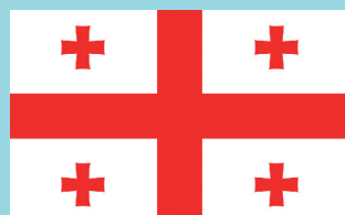
Гурджустан
