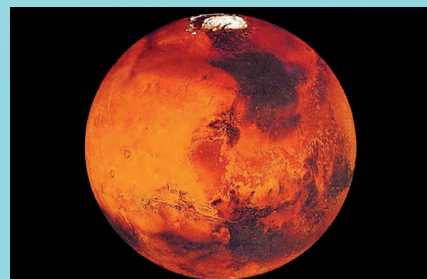
Марс
