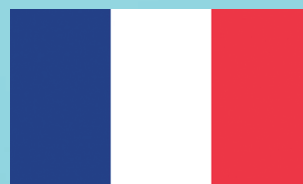
Франса
