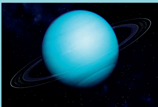
Уран
