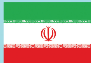
Иран
