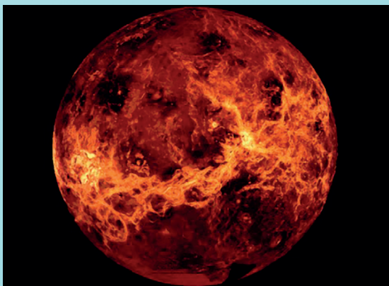
Венера
